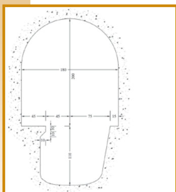
COUPE DE L'ÉMISSAIRE AVEC COTES THÉORIQUES (Dimensions exprimées en cm.)
